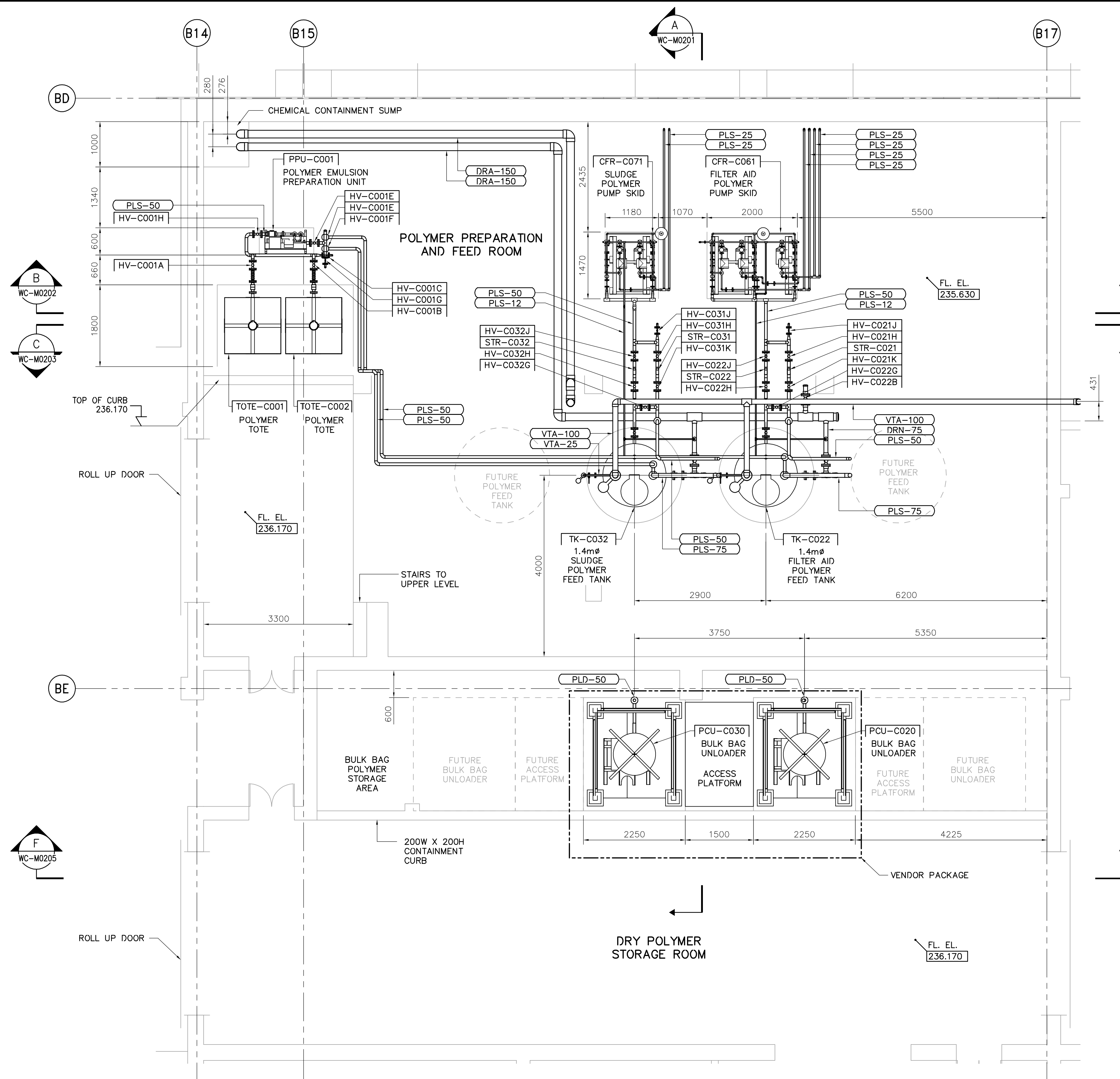
1 DETAIL WC-M0111 1:50
