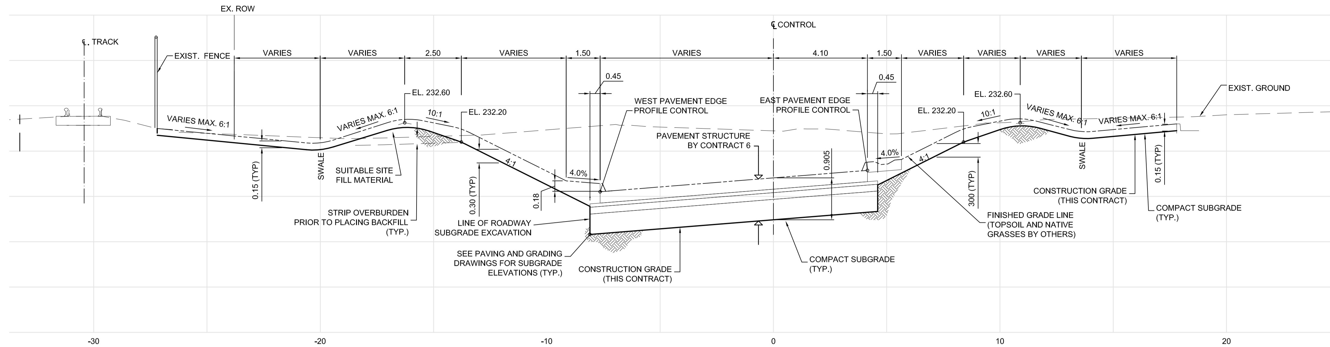
A SECTION - STA. 11+630 SCALE: H = 1:100 V = 1:50
