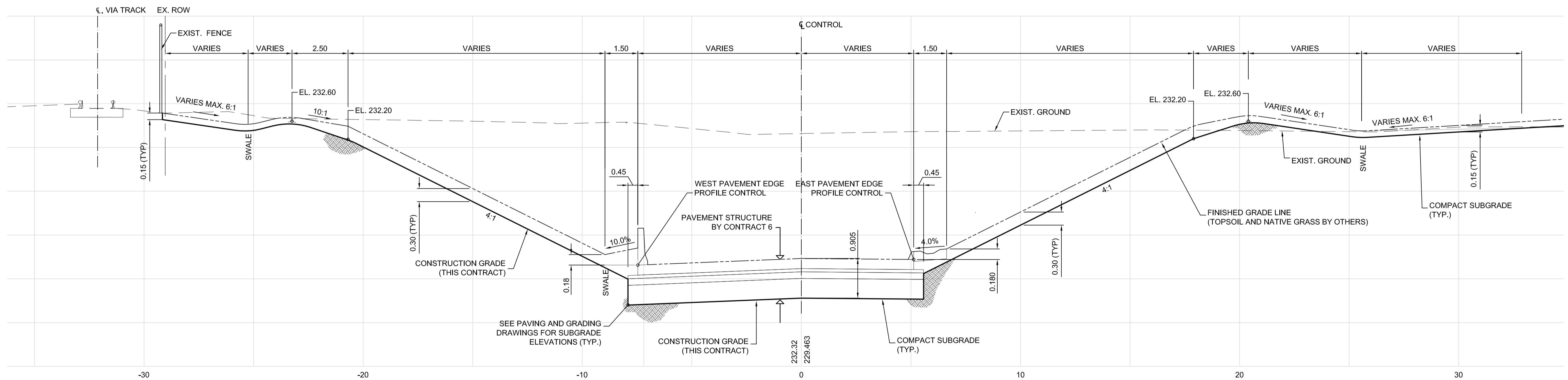
B SECTION - STA. 11+705.525 SCALE: H = 1:100 V = 1:50
