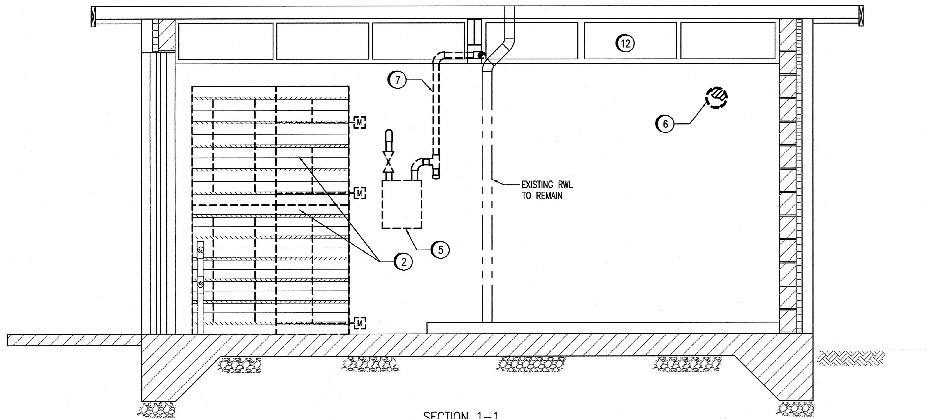
SECTION 1-1 1:20
