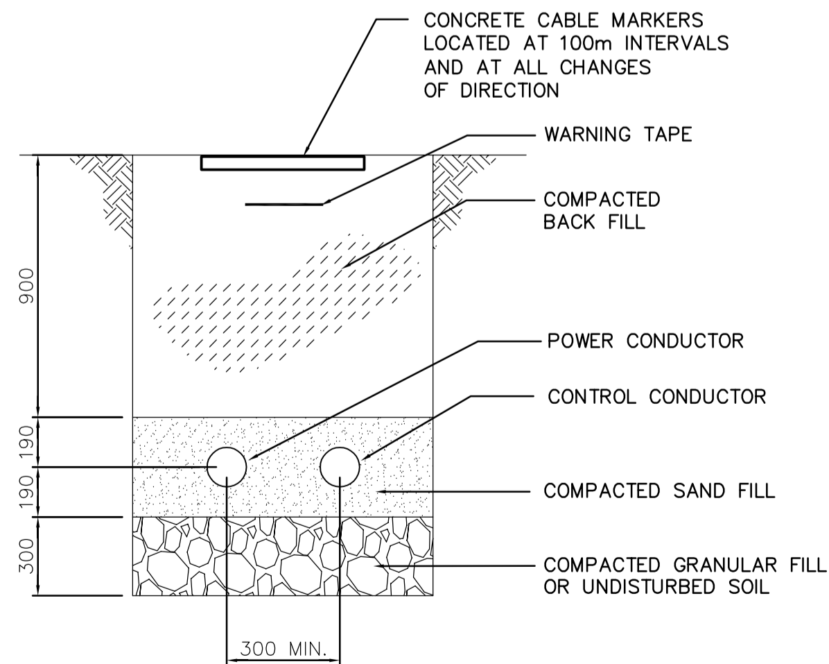
1 SECTION - CABLE TRENCH N.T.S.
