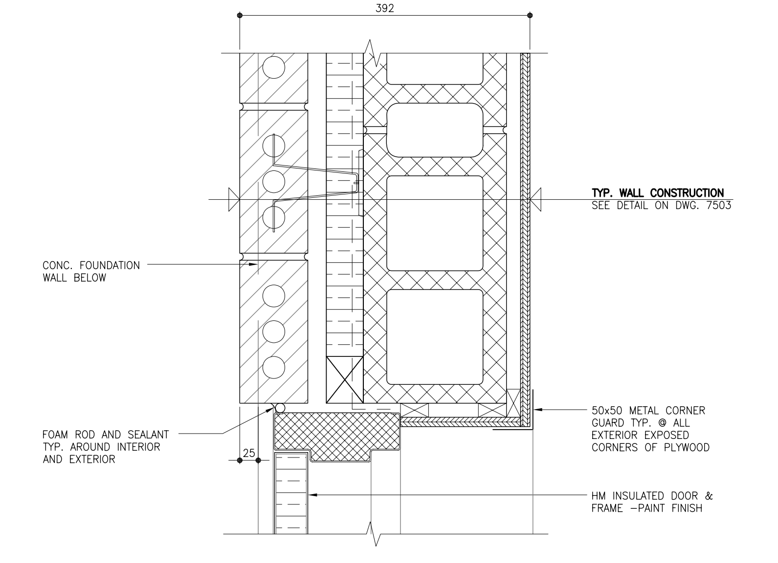
A JAMB DETAIL B04 1:5
