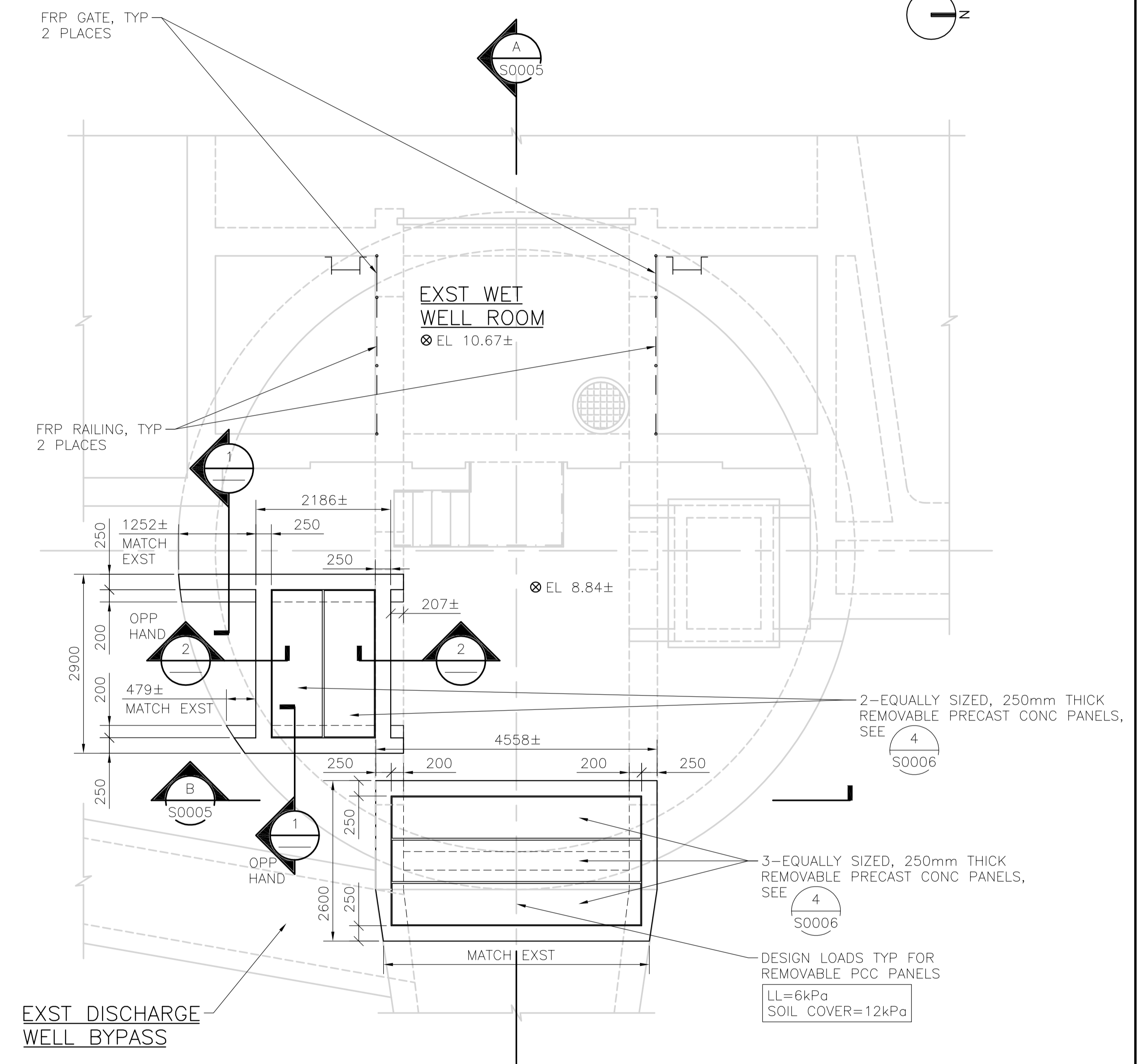
UPPER LEVEL PLAN ABOVE EL 10.67± 1:50
