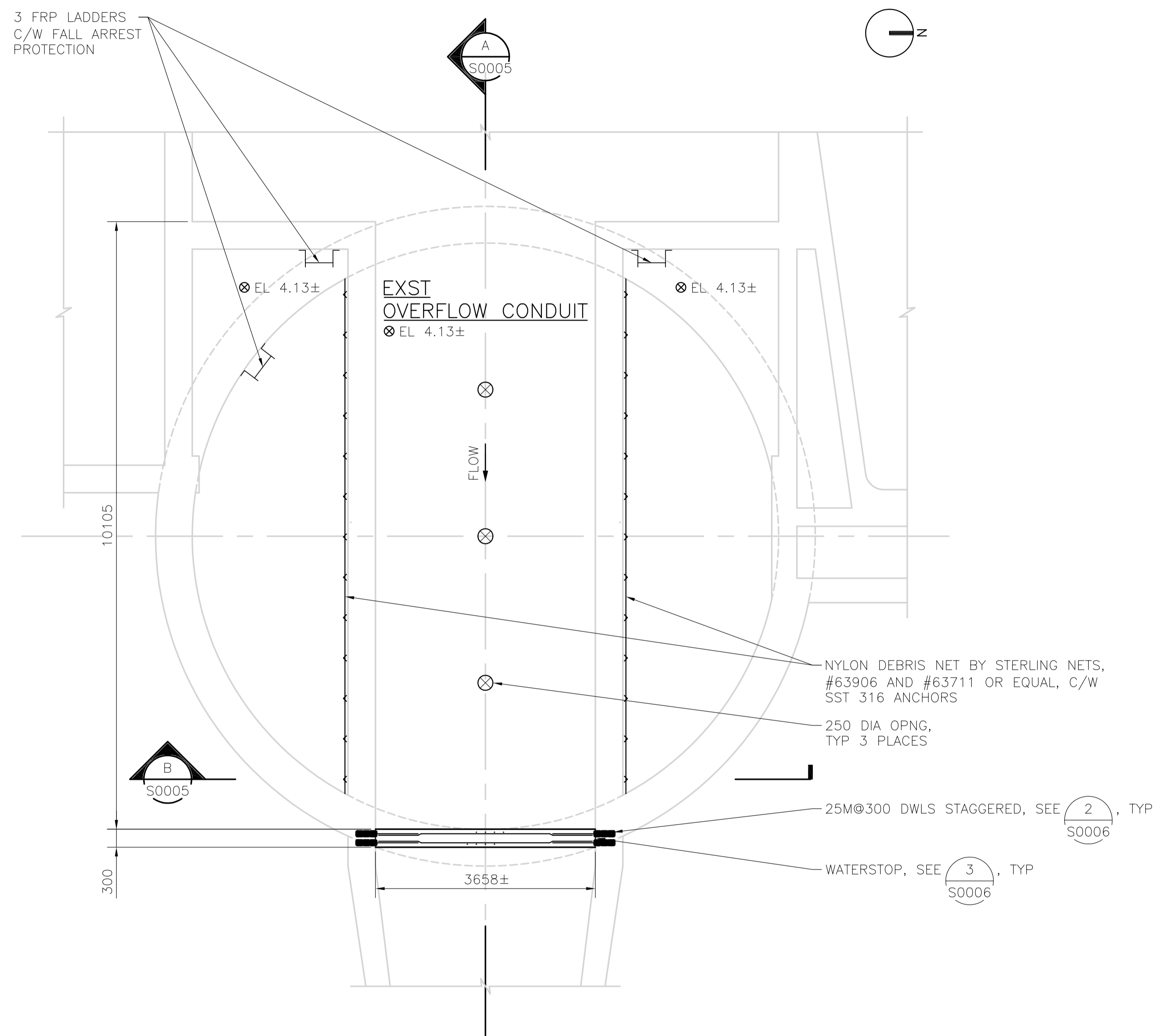
UPPER LEVEL PLAN ABOVE EL 4.13± 1:50
