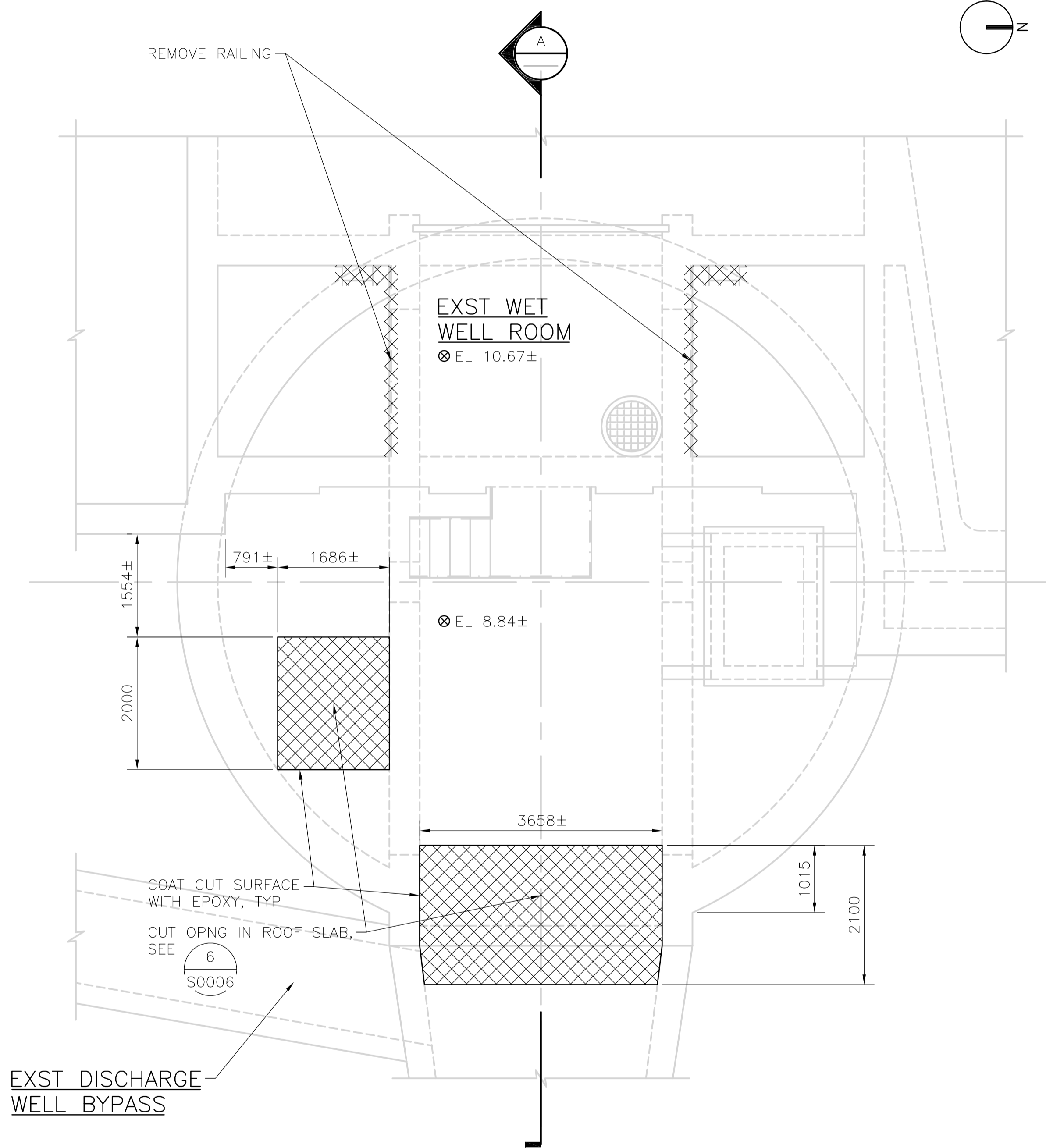
UPPER LEVEL PLAN ABOVE EL 10.67± 1:50
