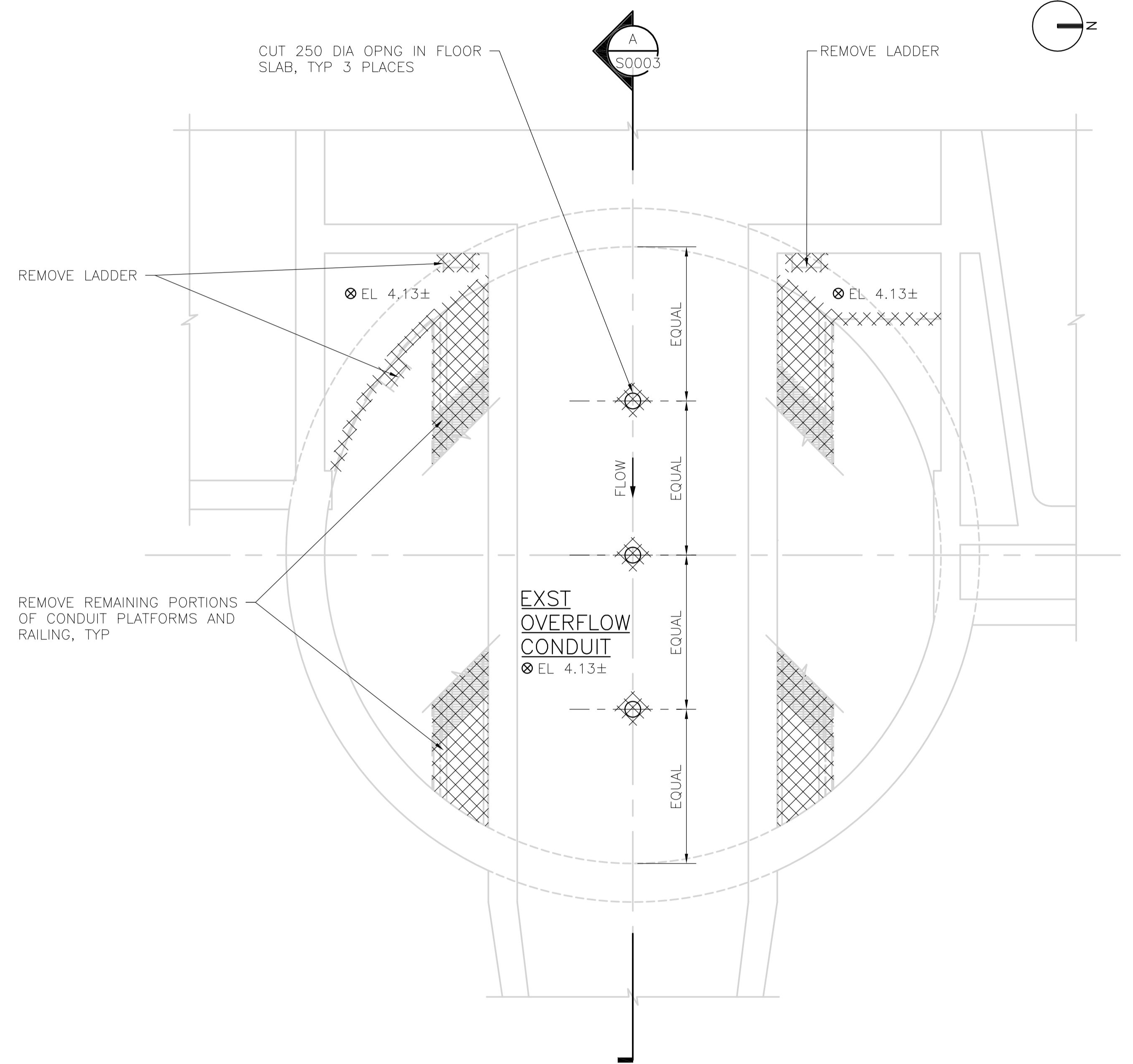
UPPER LEVEL PLAN ABOVE EL 4.13± 1:50
