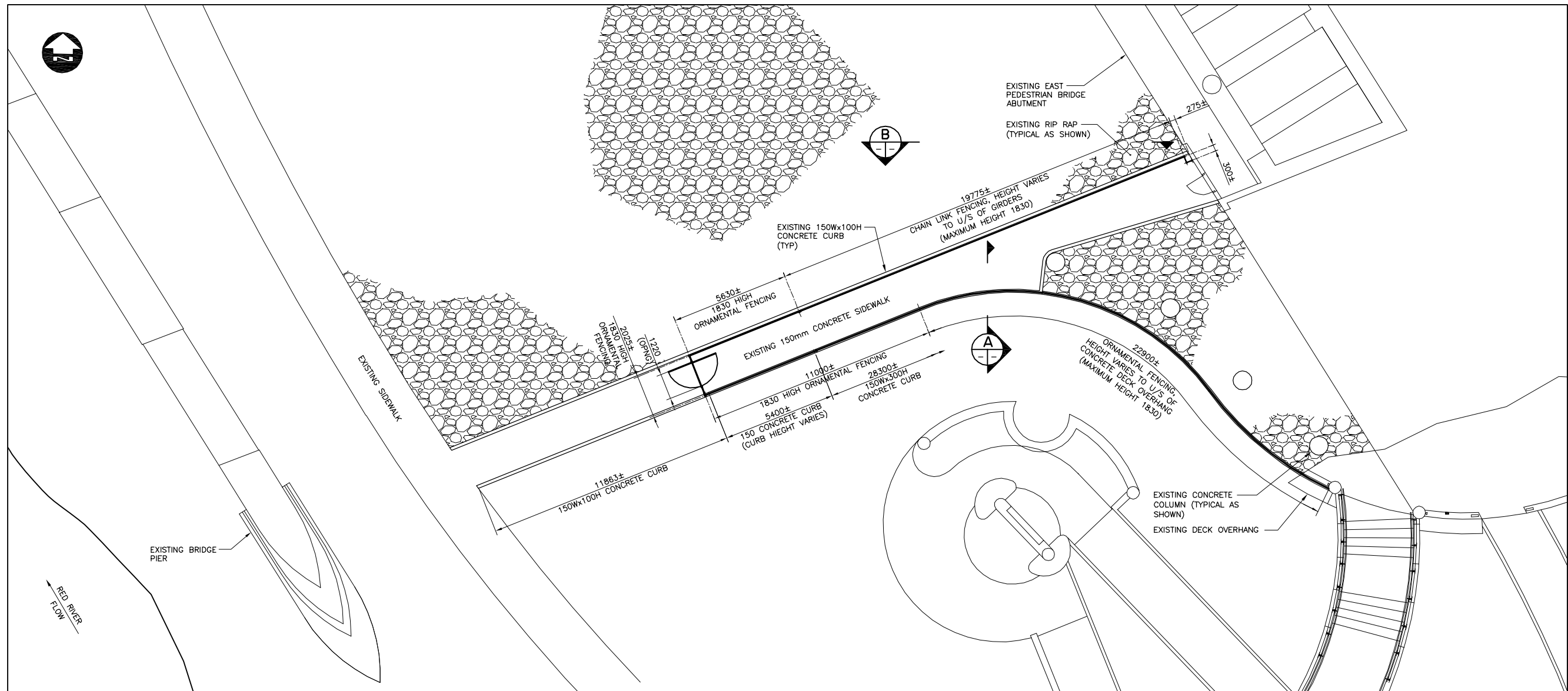
SITE PLAN 1:100
