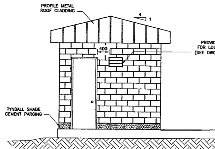
NORTH ELEVATION SCALE: 1:40
