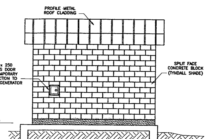
EAST ELEVATION SCALE: 1:40
