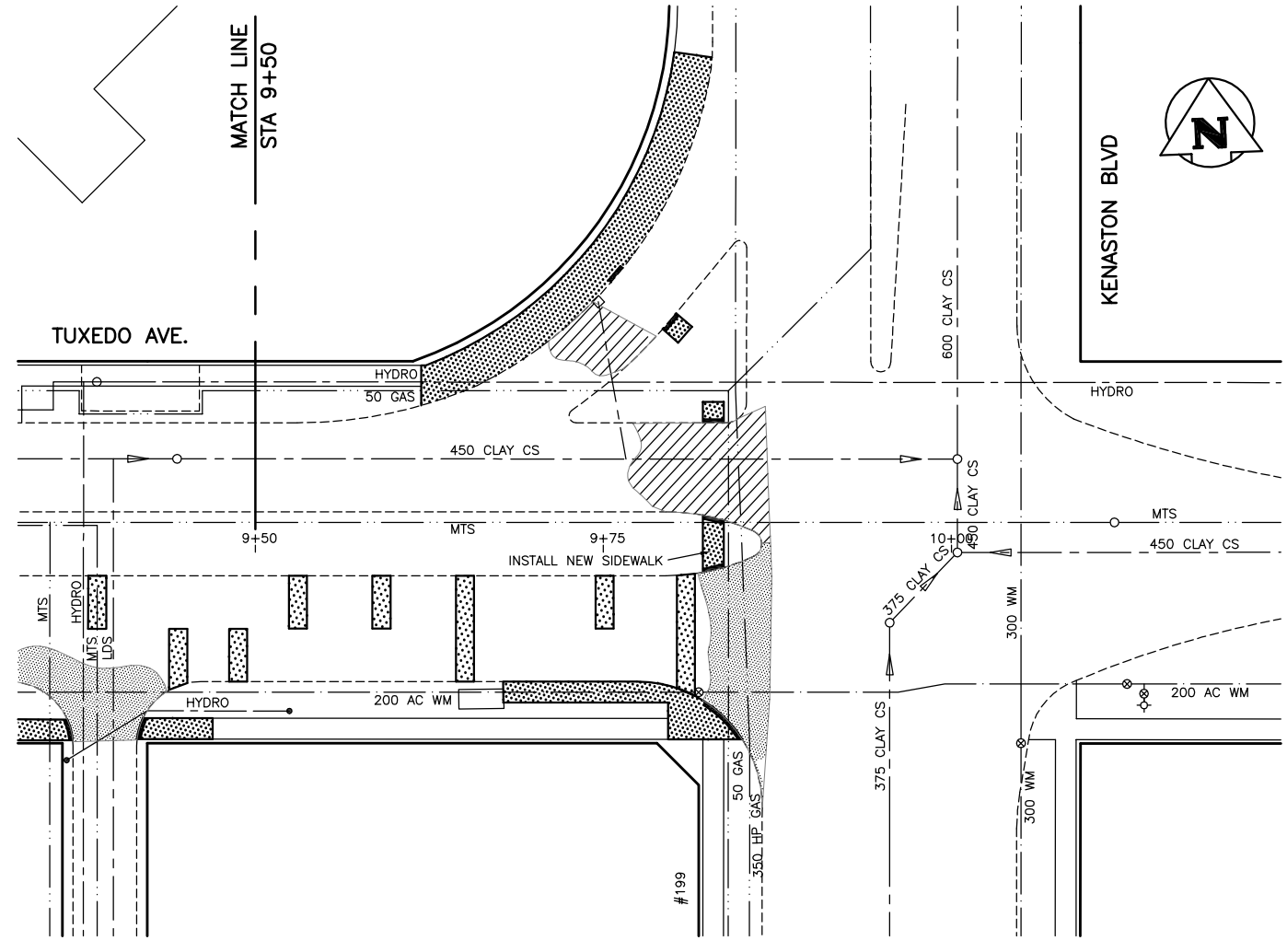
PLAN SCALE: 1:250
