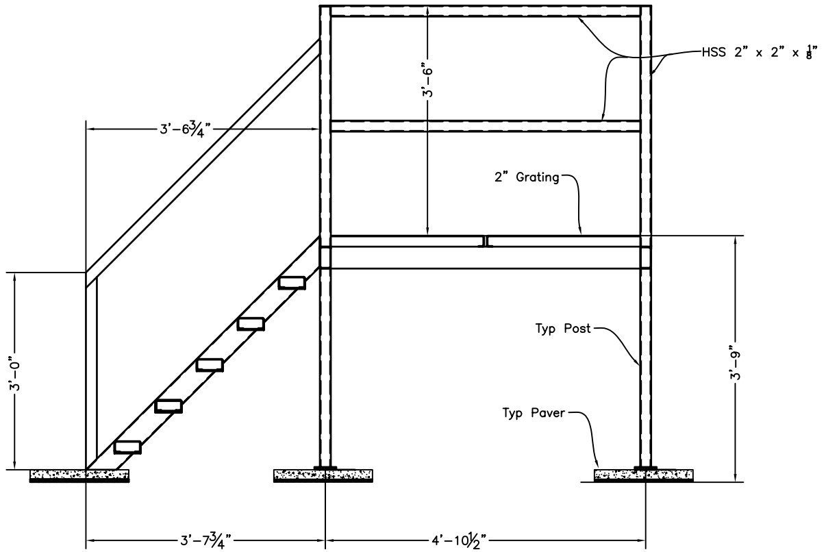
Side Elevation Scale: 1/2" = 1'-0"
