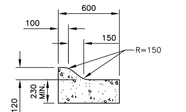
MOUNTABLE CURB & GUTTER N.T.S.
