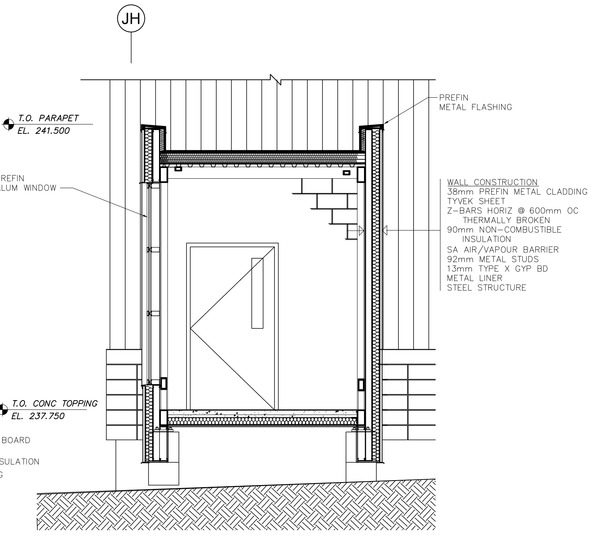
3 SECTION B WJ-B0403 1:30
