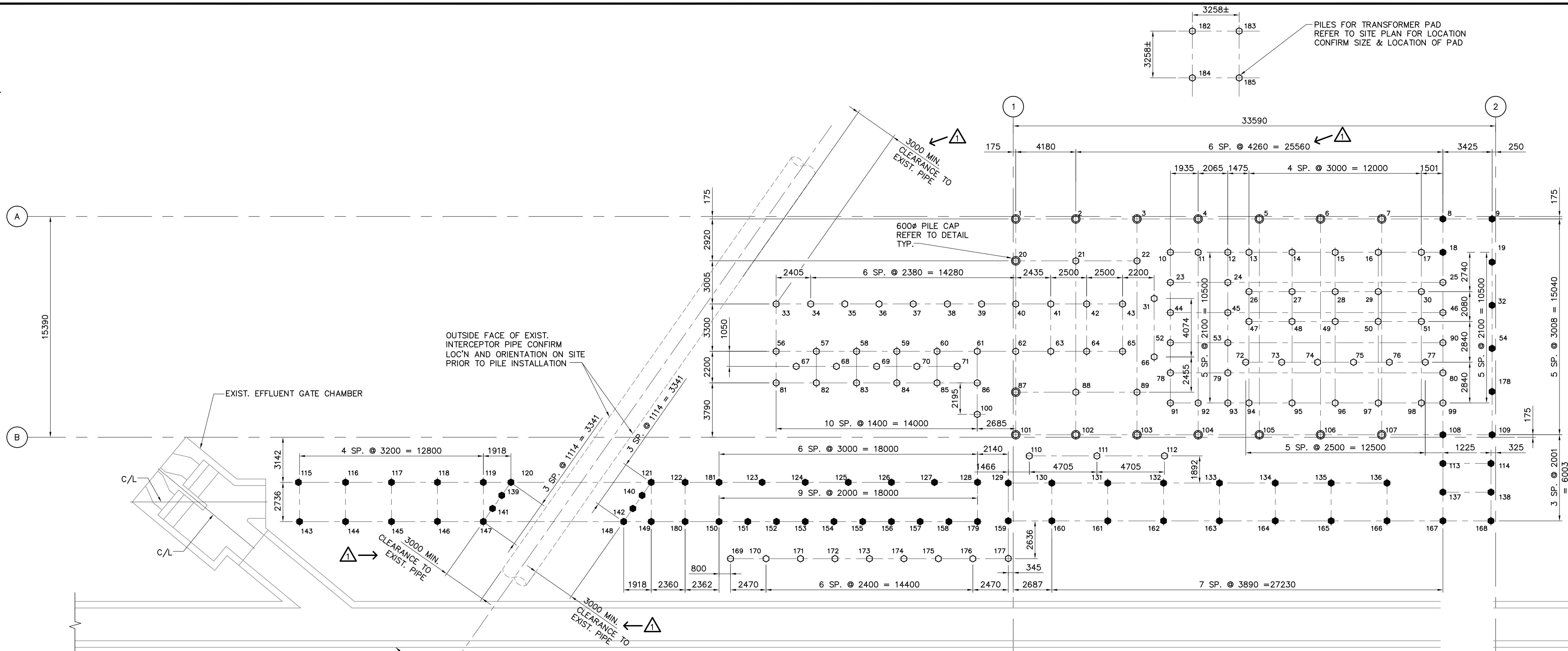
PILING PLAN SCALE: 1:150
