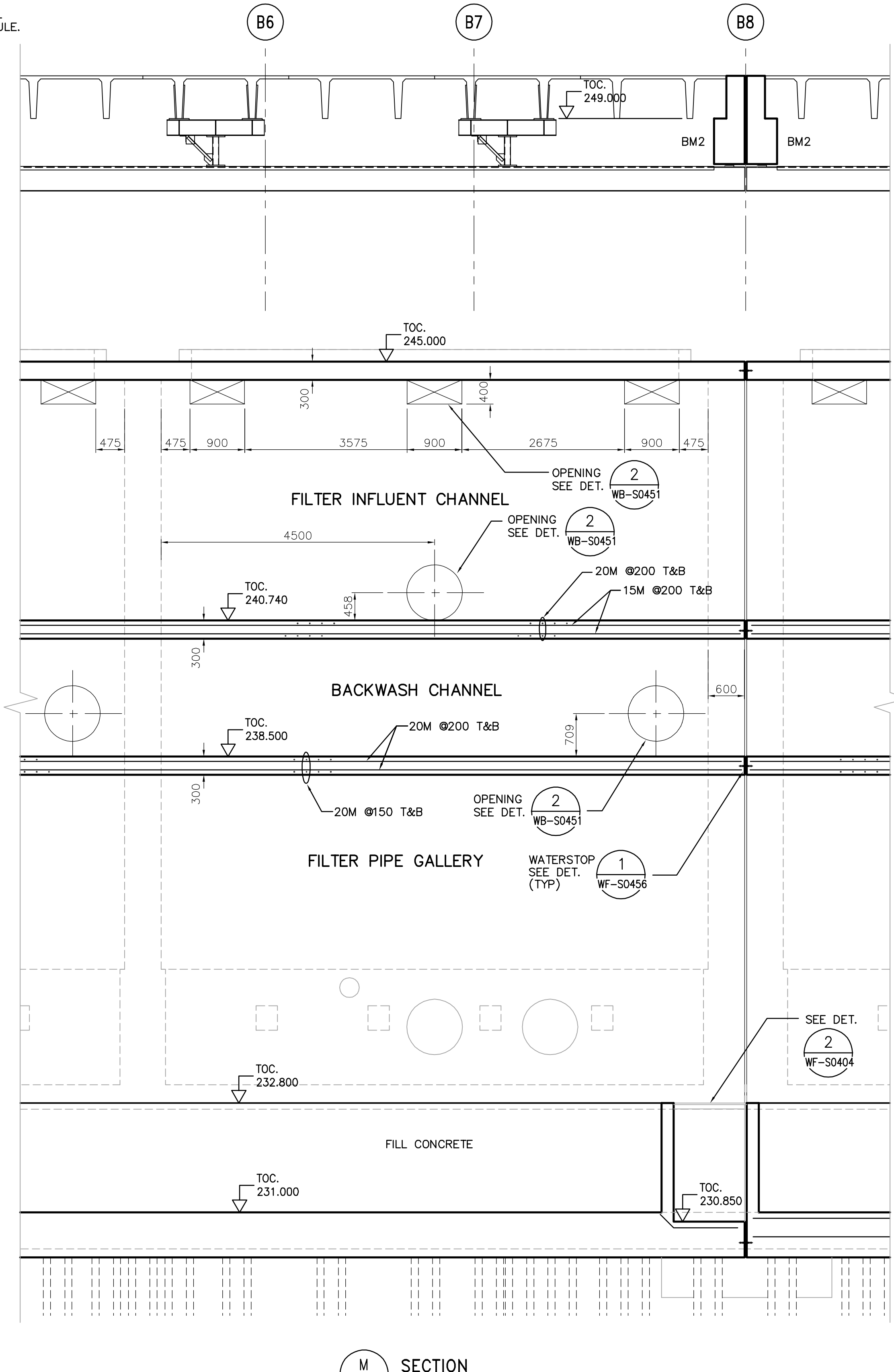
M SECTION WF-S0101 1:50 WF-S0105 WF-S0125 WF-S0111 WF-S0131 WF-S0115 WF-S0135 WF-S0117 WF-S0141 WF-S0121 WF-S0146
