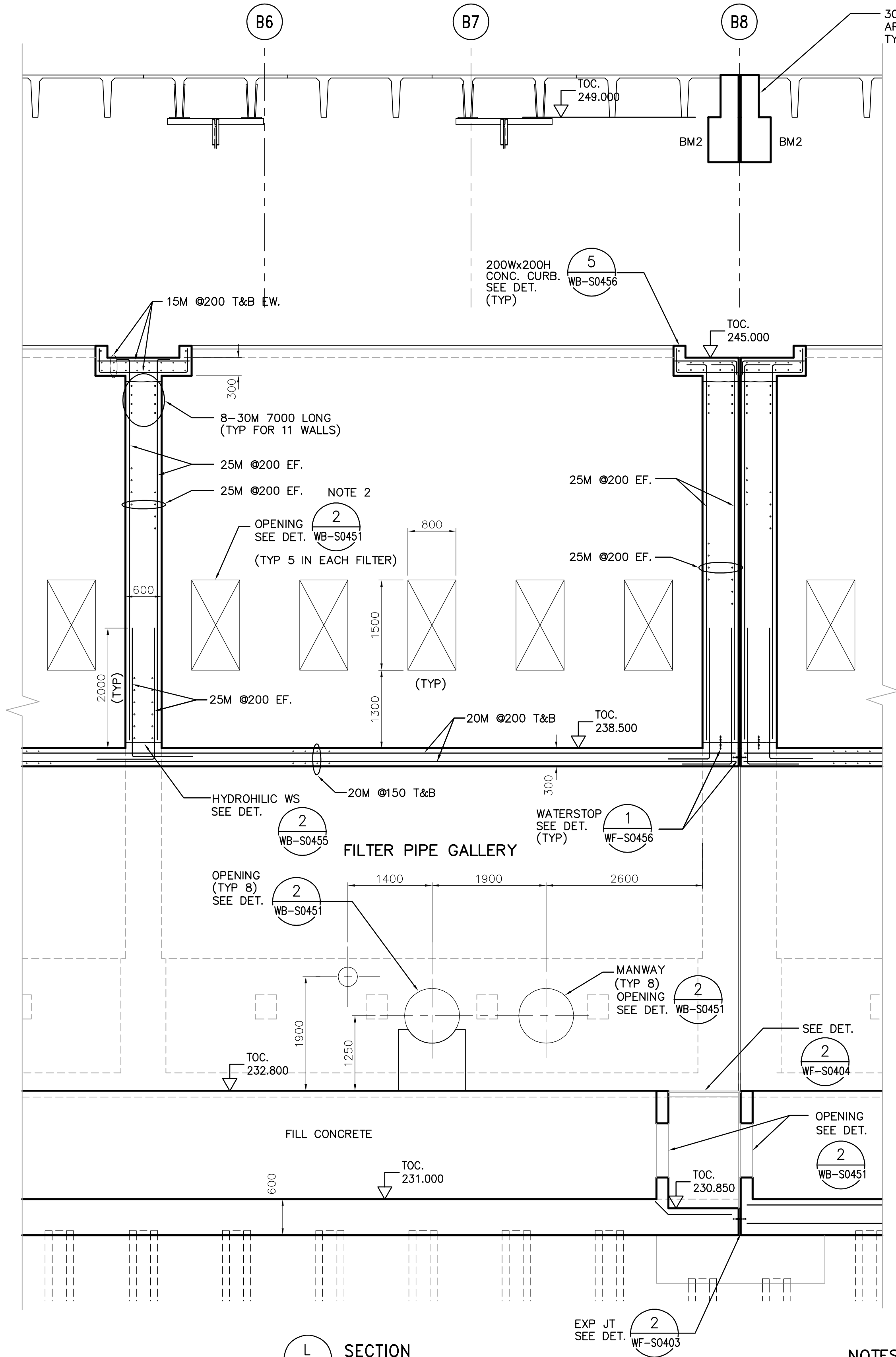
L SECTION WF-S0101 1:50 WF-S0105 WF-S0125 WF-S0111 WF-S0131 WF-S0115 WF-S0135 WF-S0117 WF-S0141 WF-S0121 WF-S0146
