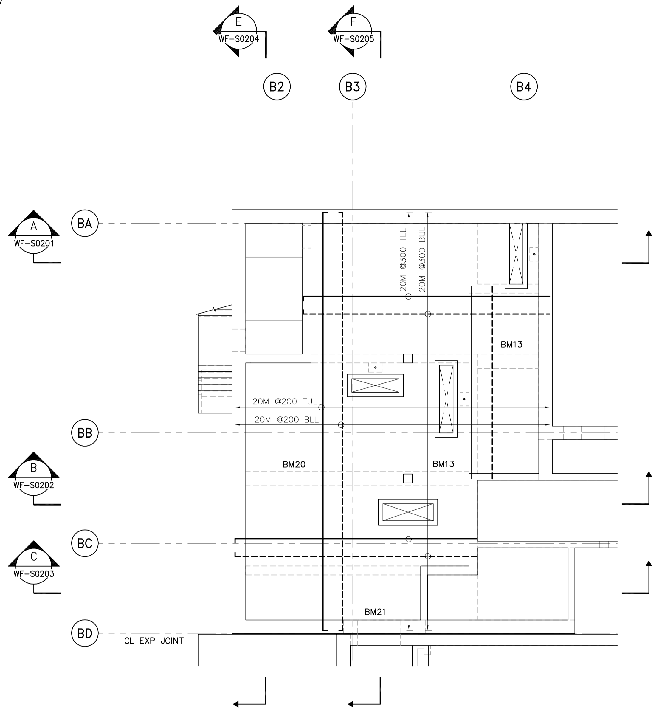
PLAN AT EL 239.410 1:100
