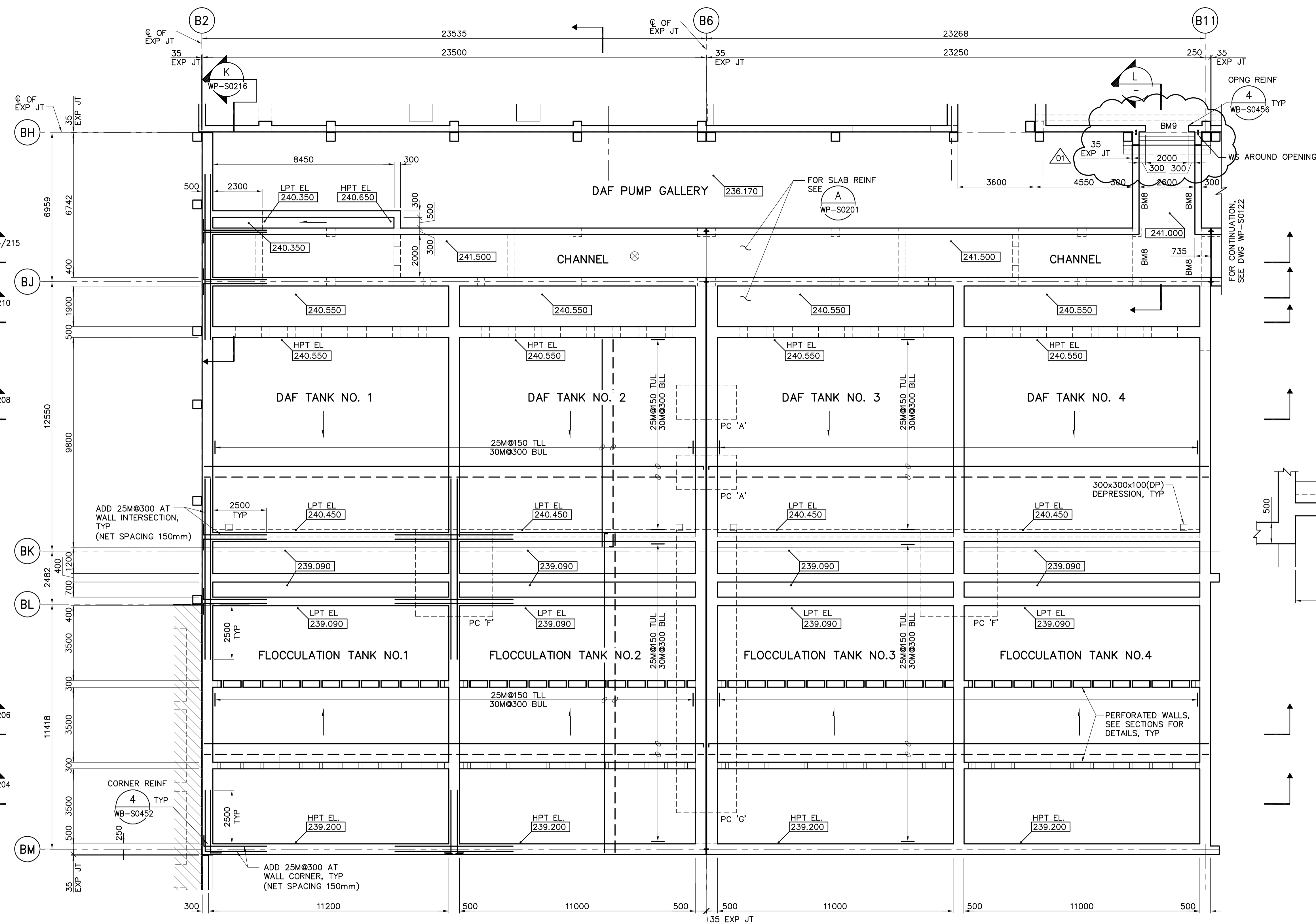
SECTION L 1:50
