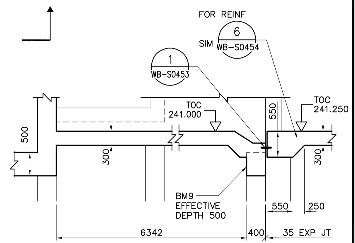
SECTION L 1:50
