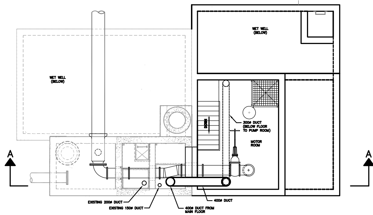
PLAN VIEW SCALE: 1:50
