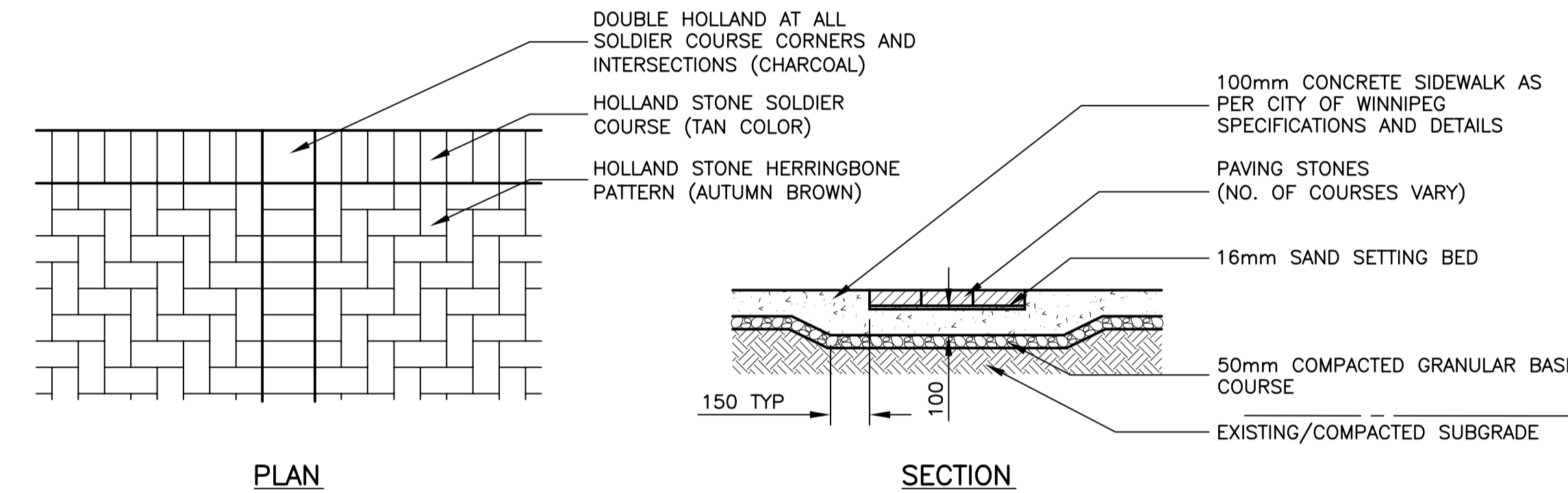
PAVING STONE DETAIL N.T.S.
