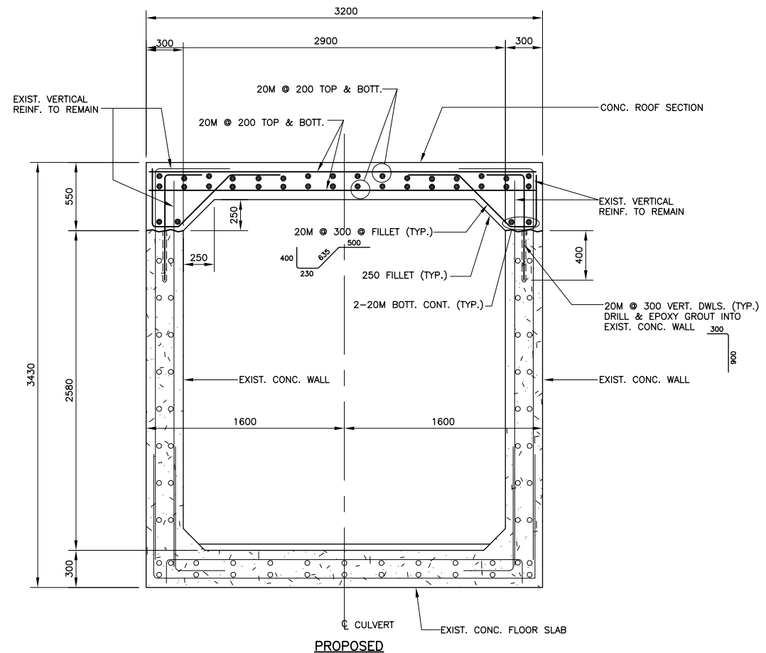
SECTION 6 1:20
