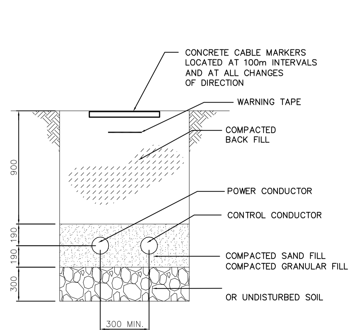
1 SECTION - CABLE TRENCH N.T.S.
