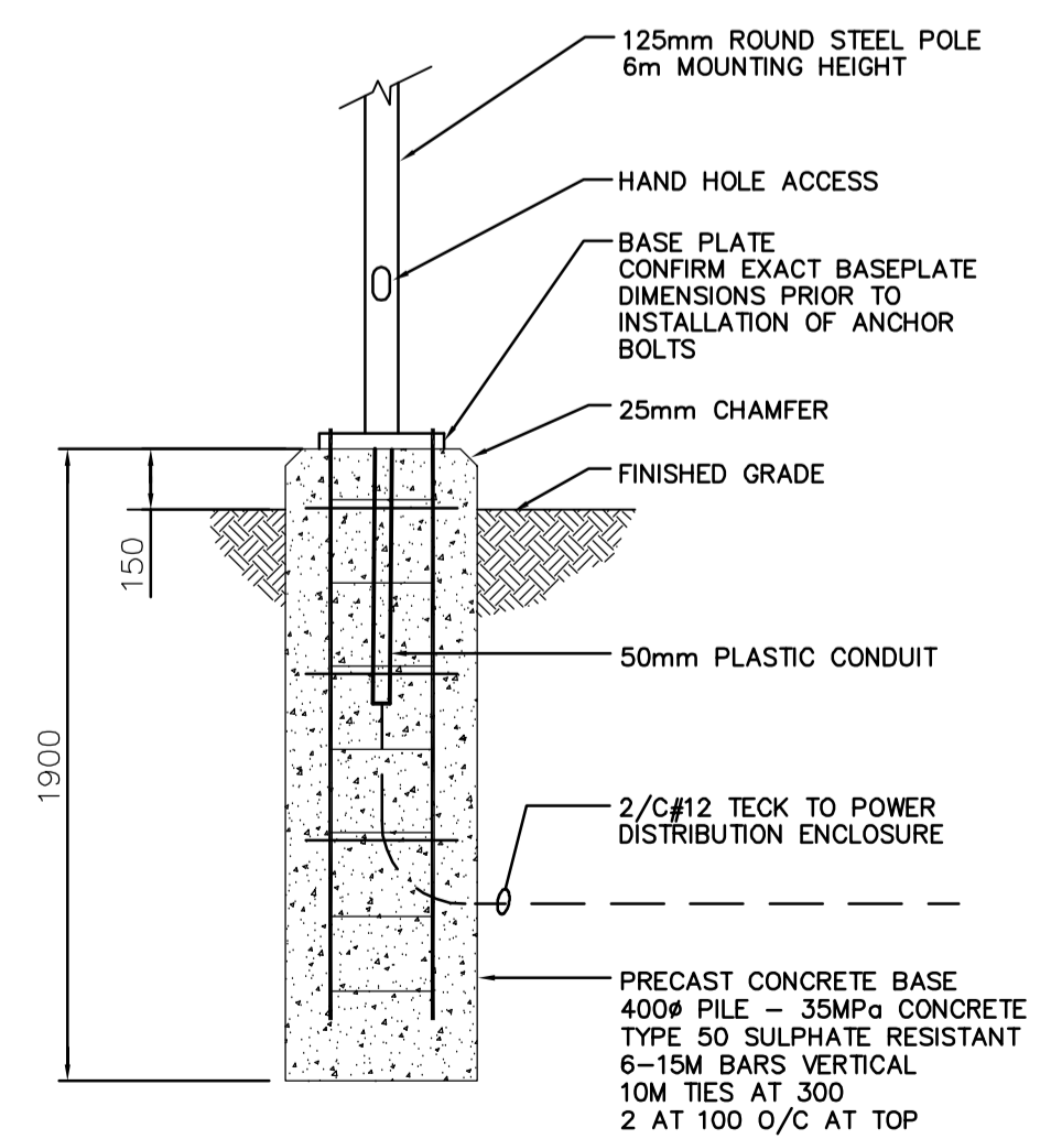
F DETAIL - POLE BASE N.T.S.
