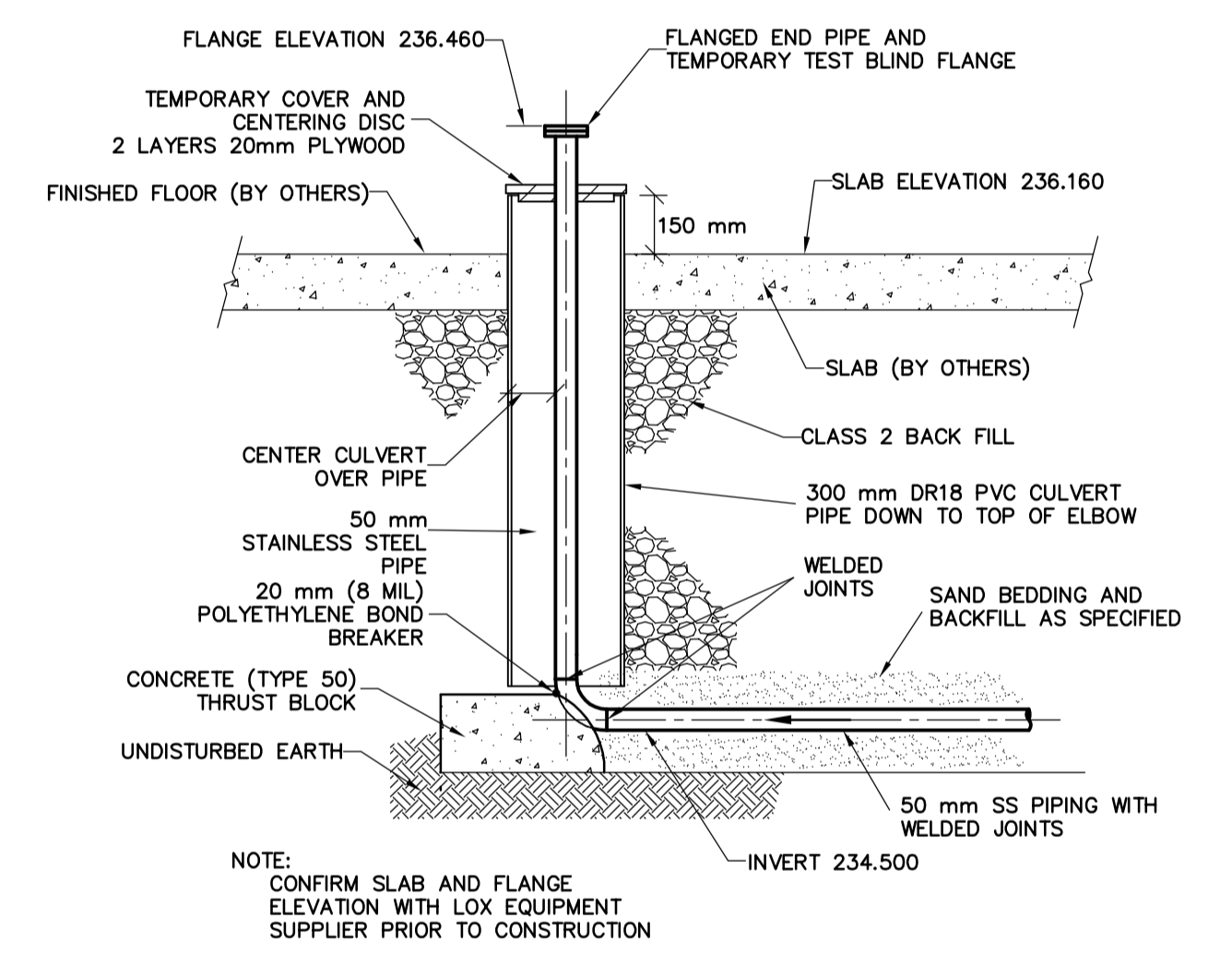
1 GOX PIPING RISER DETAIL SCALE N.T.S.
