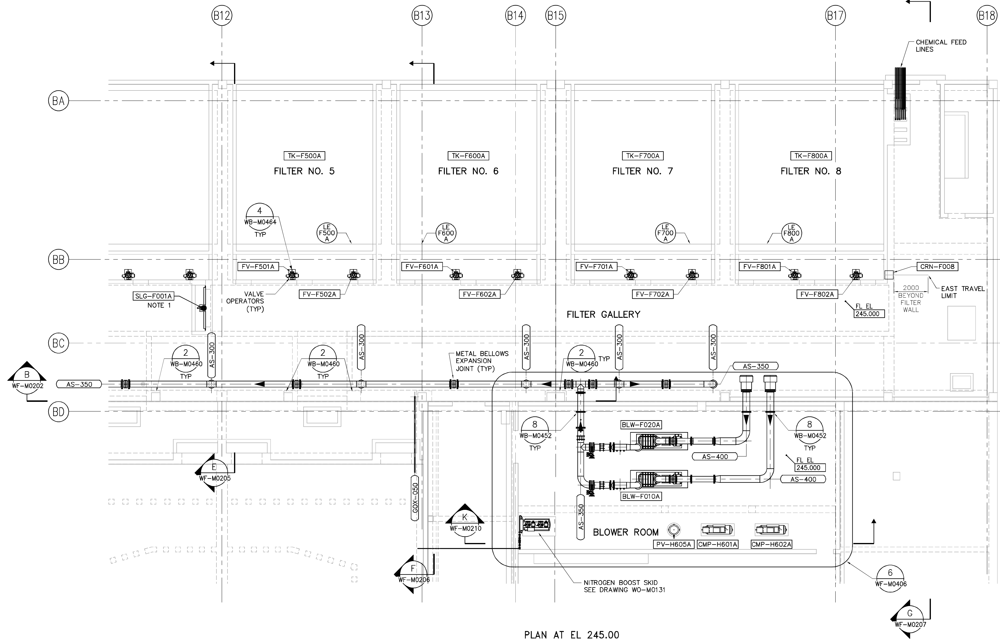
PLAN AT EL 245.00 1:100
