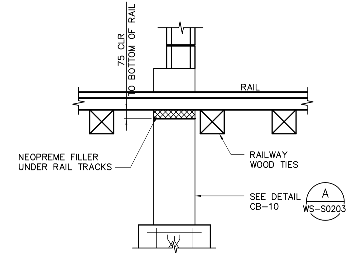
1 SECTION WS-S0203 1:20
