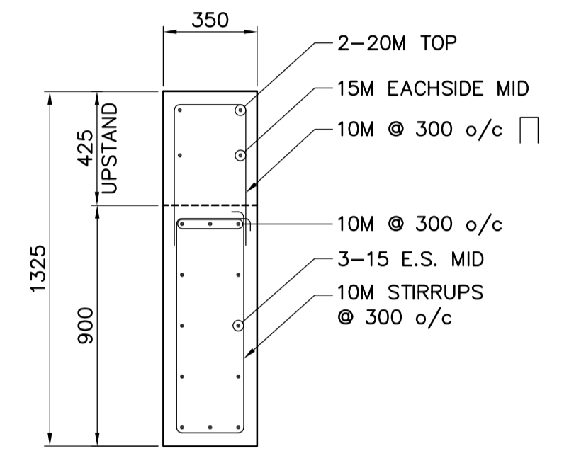
A CB-10 DETAIL WS-S0203 1:20
