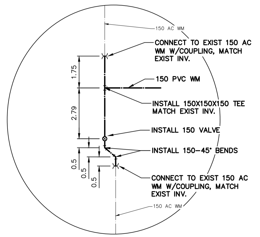
DETAIL "A" SCALE N.T.S.
